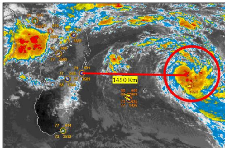
Meteosat IODC du 14/01/2018 à 09 heures locales
